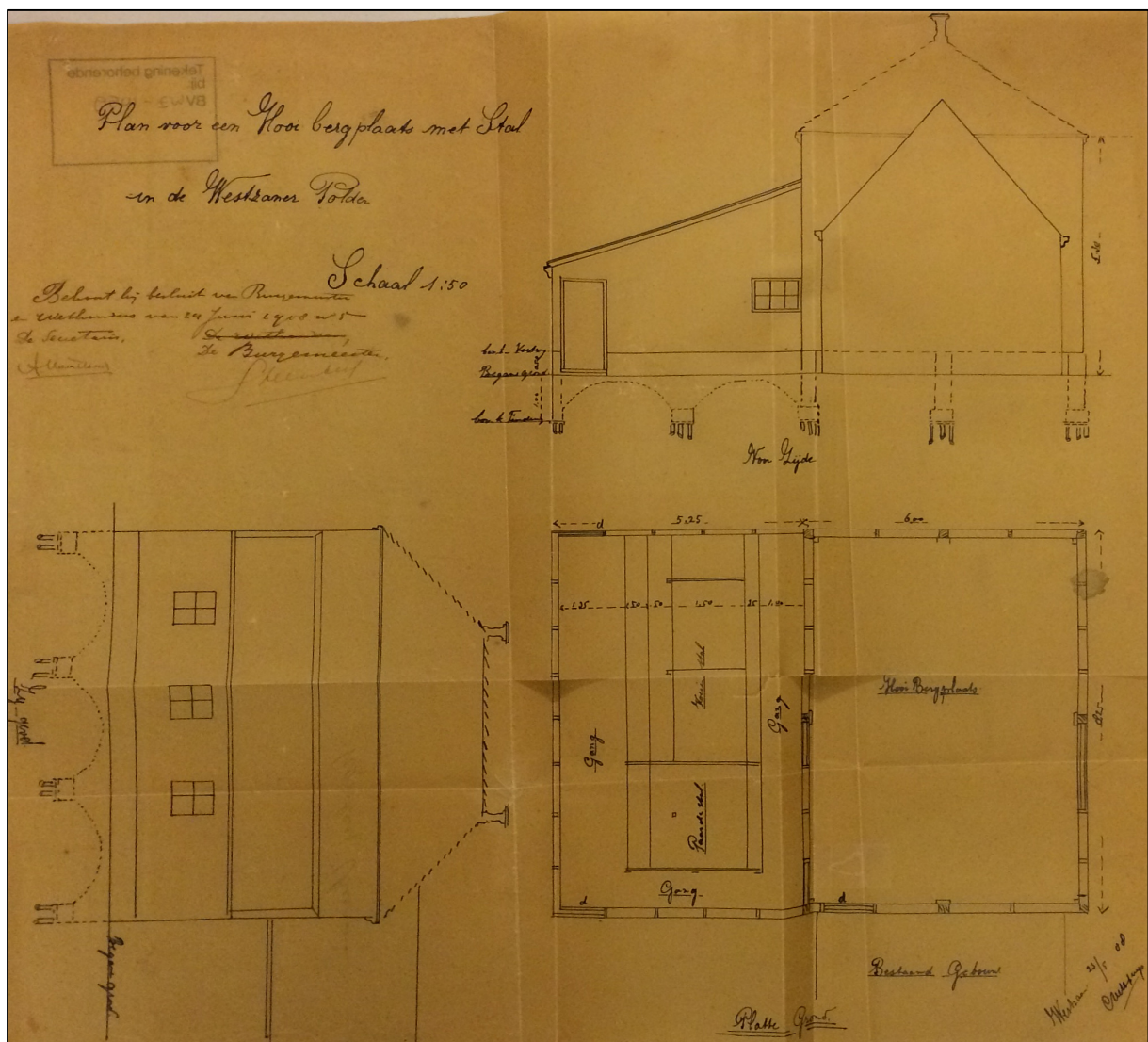
Bouwtekening van een huis en hooiberg uit 1908 op Overtoom 79, voor het ouderlijk huis Veldweg 255, omstreeks 1922 aangekocht door Gerrit Heermans. Foto © Bouwtekening collectie Gemeentearchief Zaanstad.
