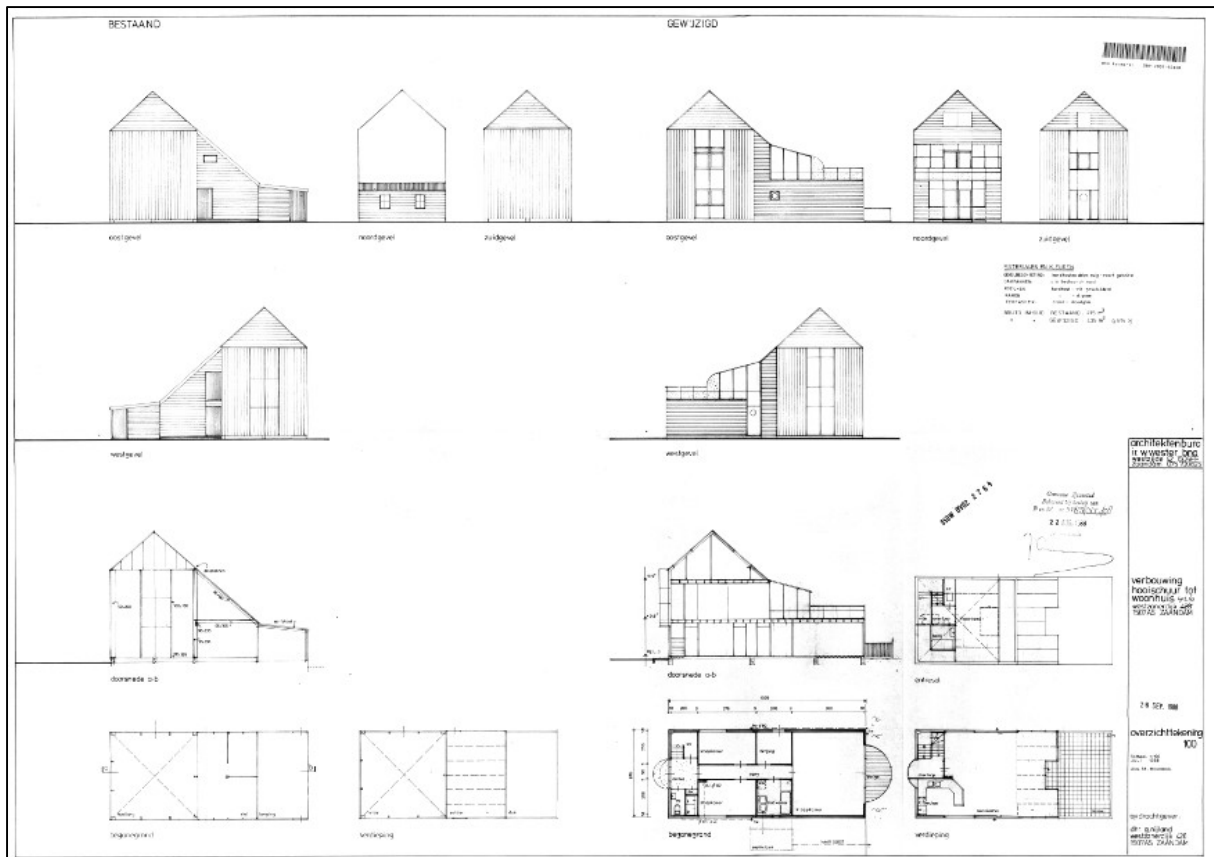
Bouwtekening voor de verbouw van de hooiberg uit 1928 tot woning Westzanerdijk 426.
