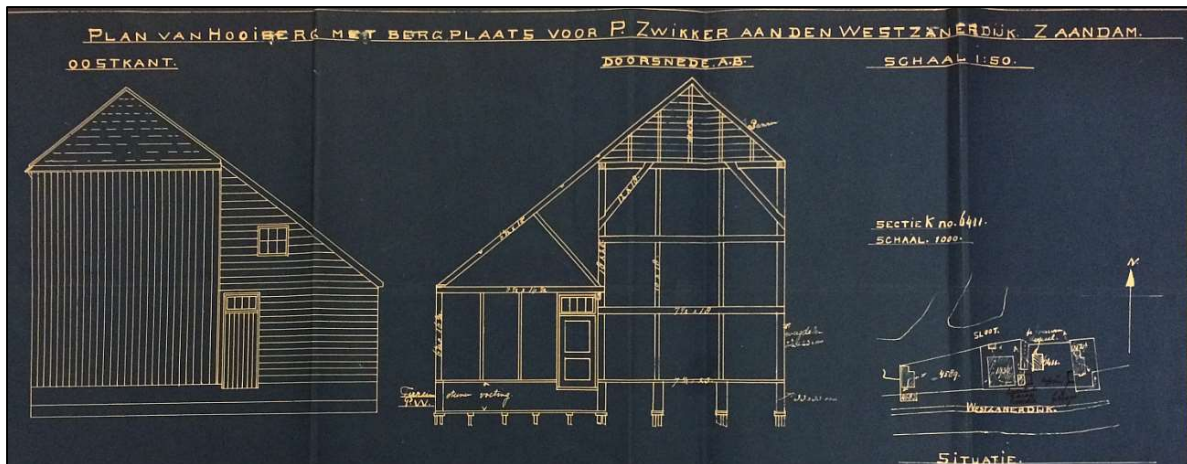
Bouwtekening voor de hooiberg bij de boerderij Westzanerdijk 428, gebouwd in 1928.
