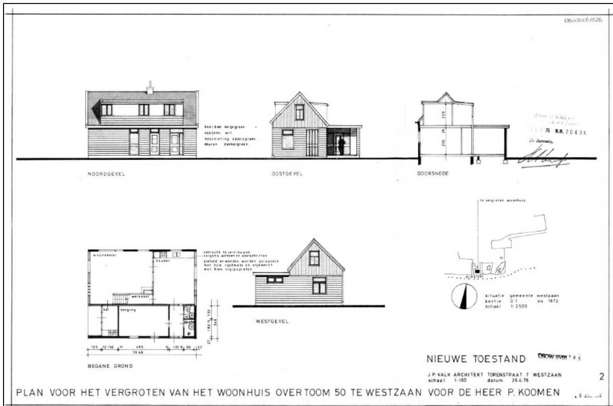
Bouwtekening van de vergroting van het woonhuis Overtoom 50 (minimaal van voor 1827) in 1978 door Piet Koomen.
