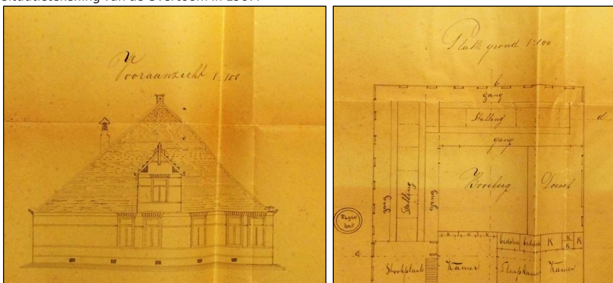
Delen van de bouwtekening in 1907.
