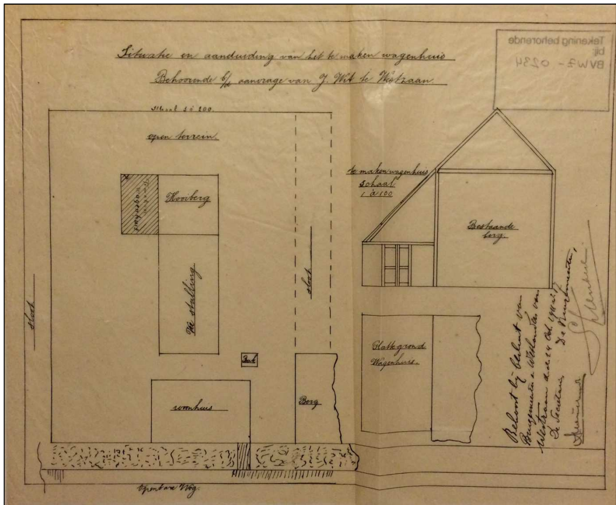
De bouwtekening van de wagenloods achter de boerderij in 1911, aan de stal en hooiberg uit 1906. © Collectie Gemeentearchief Zaanstad.
