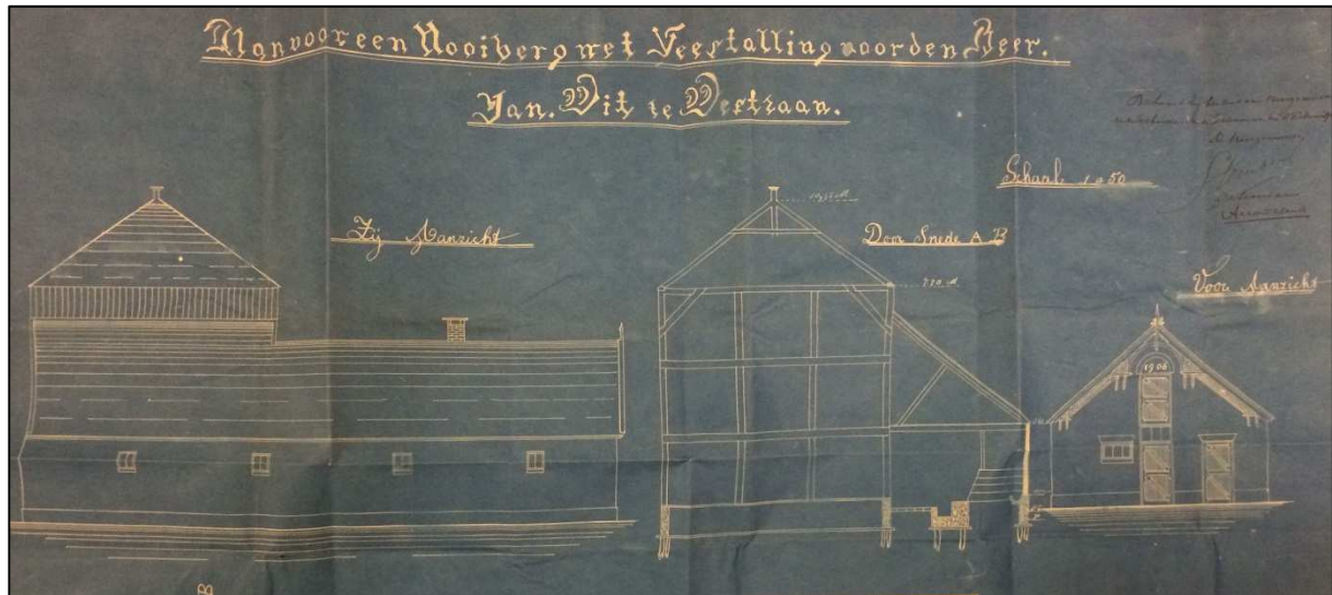
Bouwtekening van de stal en hooiberg uit 1906, op de plek van een stal uit 1879, achter het woonhuis uit 1868. In werkelijkheid werden deze iets anders uitgevoerd. © Collectie Gemeentearchief Zaanstad.
