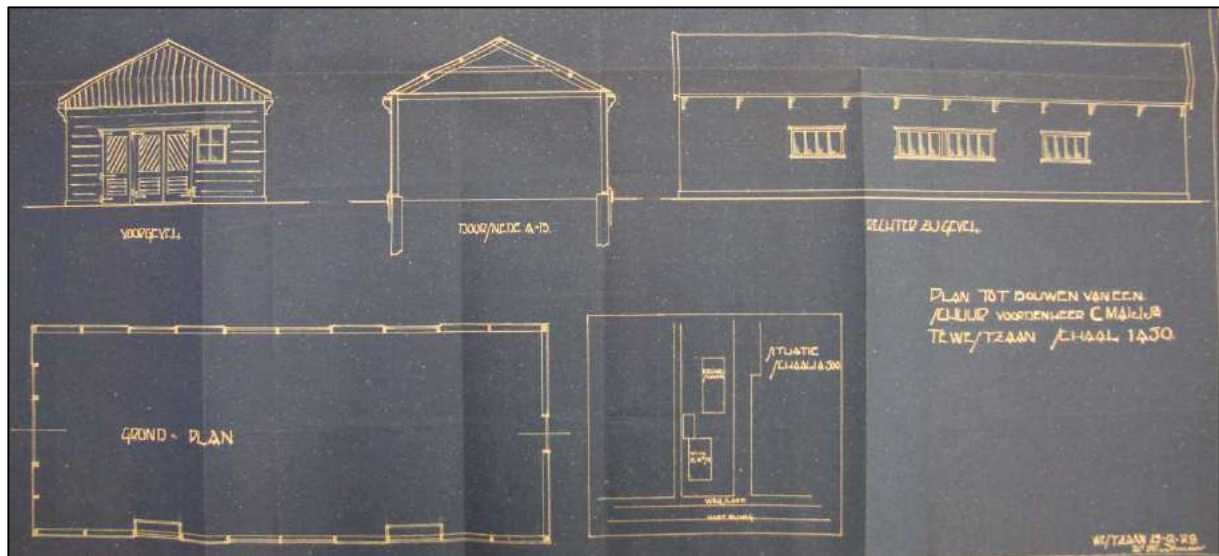
Bouwtekening van de schuur uit 1930.
