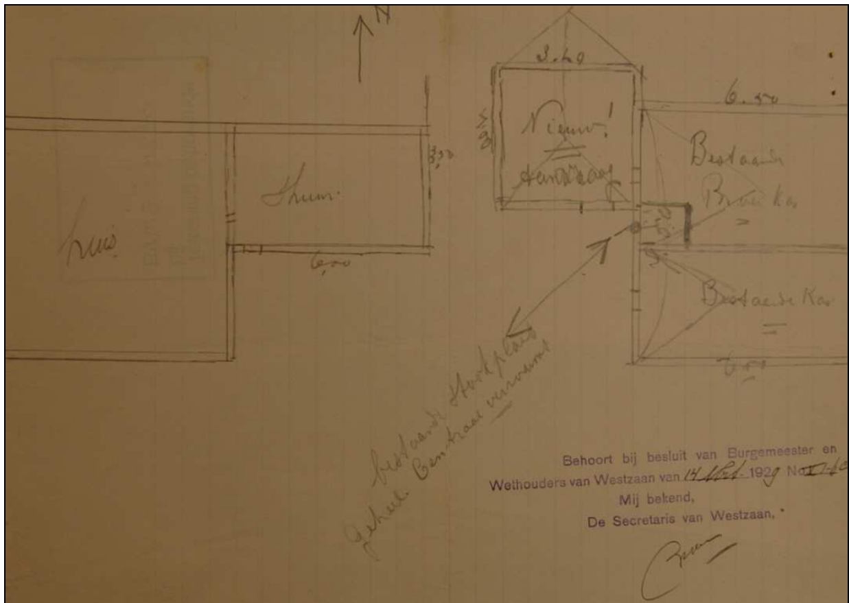
De ontwerptekening/plattegrond van de nieuwe broeikassen van Gerrit Tanger achter zijn huis aan de J.J. Allanstraat in 1929.
