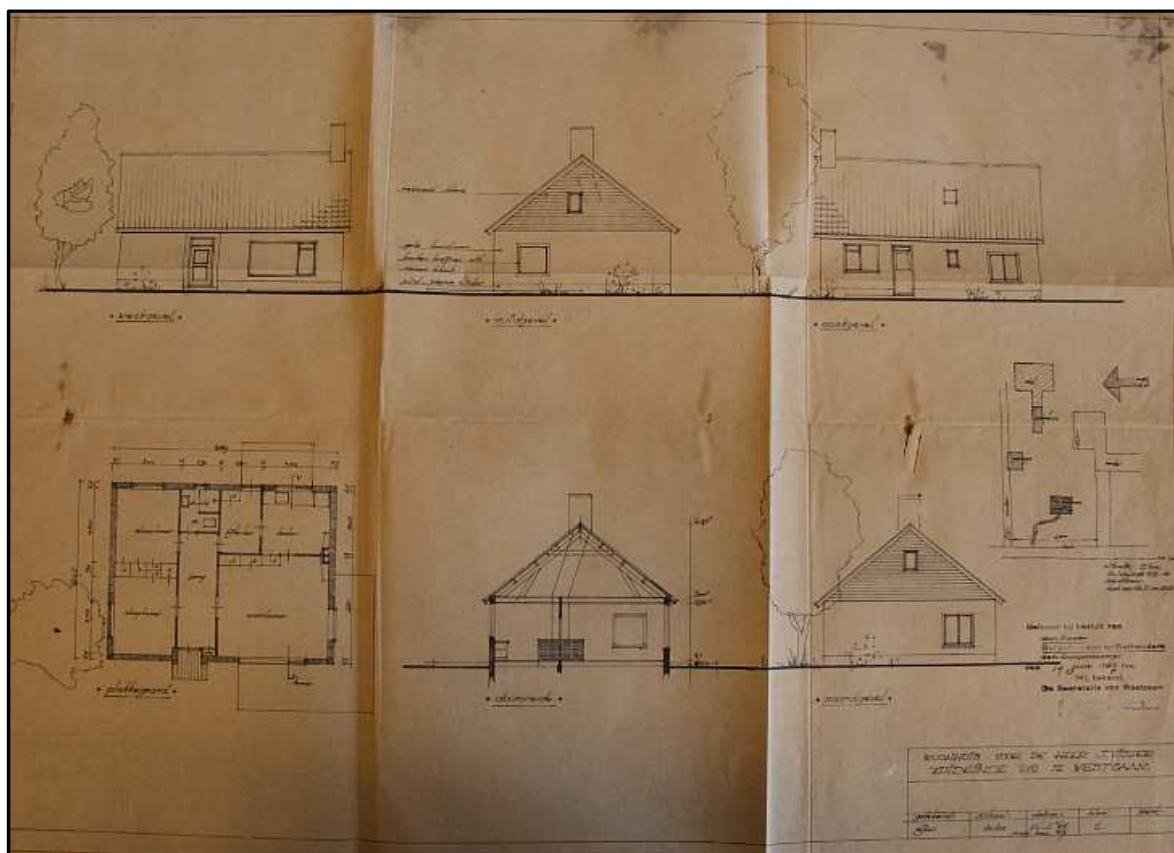
Bouwtekening van de bungalow van Jan Visser, gebouwd in 1967, Zuideinde 210.
