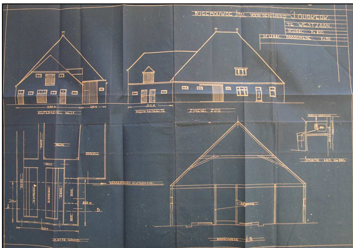
Bouwtekening van de boerderij Zuideinde 193 uit 1945 in verband met de aanbouw van een ruim acht meter lange stal.
