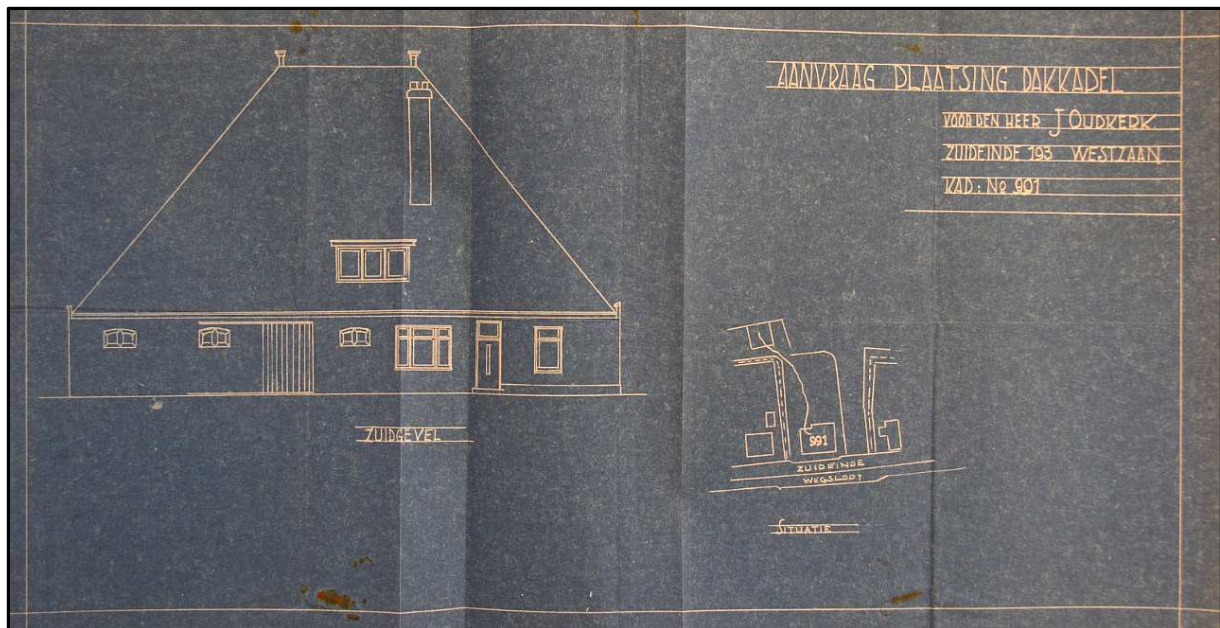
Bouwtekening van de boerderij Zuideinde 193 uit 1943 in verband met de plaatsing van een dakkapel aan de zuidzijde.
