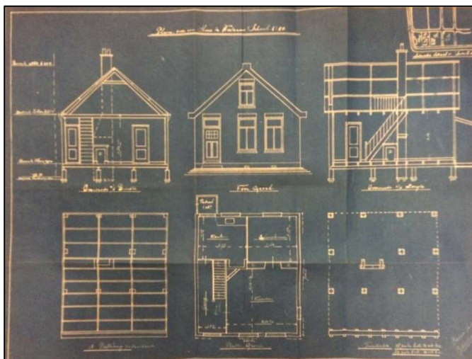
Bouwtekening van het huis van De Boer uit 1924.
